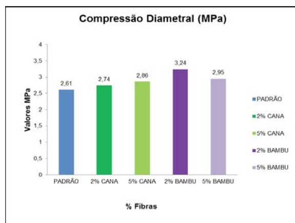
Figura 4- Dados referentes ao ensaio de resistência à tração por compressão diametral [23]
