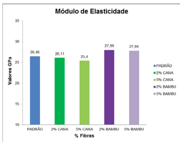
Figura 6- Dados referentes ao módulo de elasticidade estático [23]
