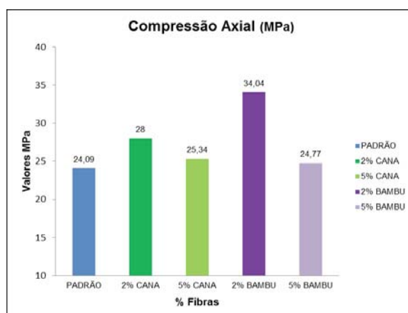
Figura 3- Dados referentes ao ensaio de resistência à compressão axial [23]
