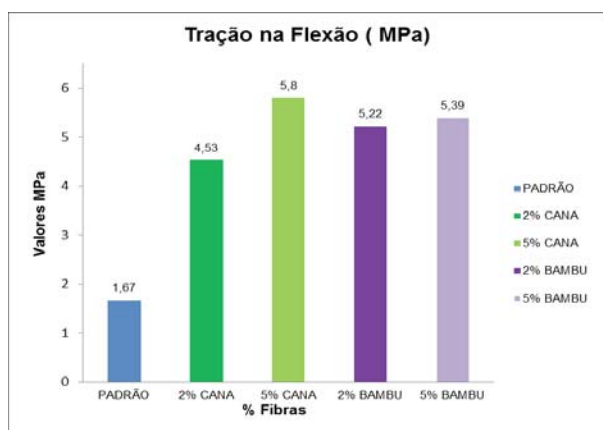
Figura 5- Dados referentes ao ensaio de resistência à tração na flexão [23]
