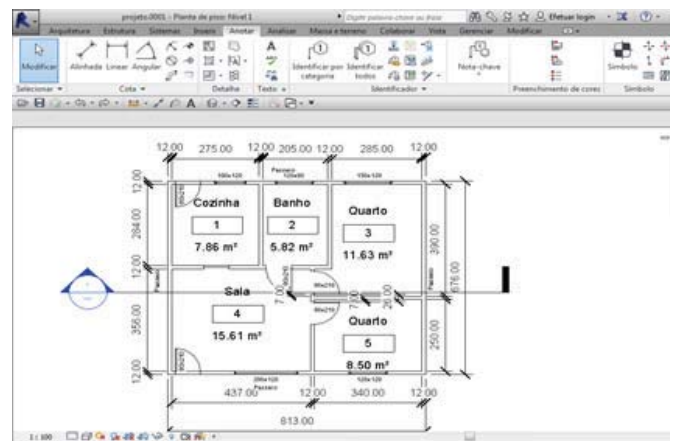
Figura 2 - Planta baixa da edificação no Revit
