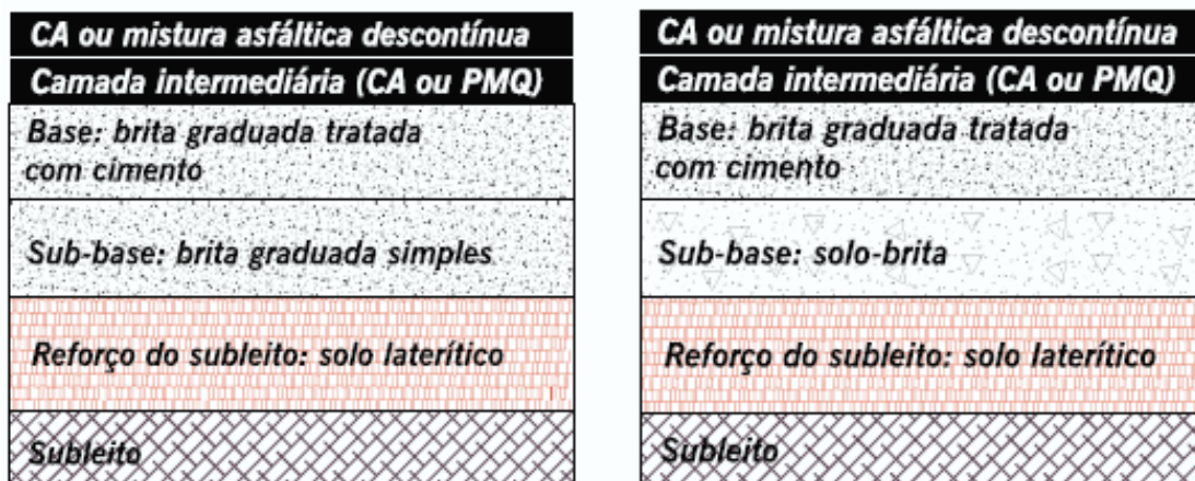
Estrutura típica de pavimentos flexíveis
