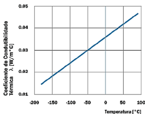
Figura 8 – Coeficiente de condutibilidade térmica do EPS de densidade 20 kg/m 3
