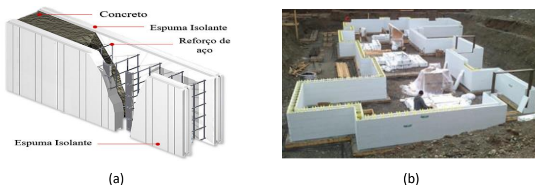
Figura 3 – (a) Bloco de EPS isolado; (b) Sistema de blocos de EPS em construção
