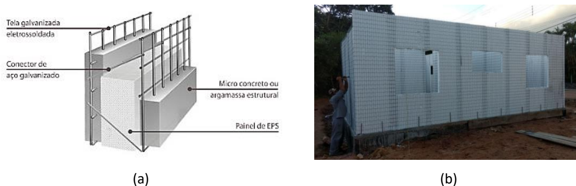
Figura 4 – (a) Painel de EPS isolado; (b) Sistema de painéis de EPS em construção
