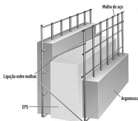
Figura 2 – Painel autoportante em EPS
