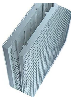
Figura 4 – Painel duplo em EPS
