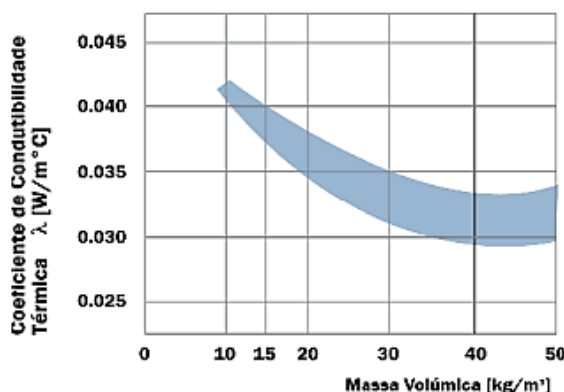
Figura 7 – Coeficiente de condutibilidade térmica do EPS
