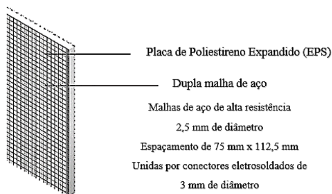
Figura 3 – Exemplo de painel simples em EPS
